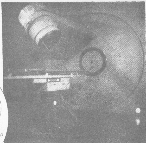
医用电子直线加速器 BJ—10 外貌
