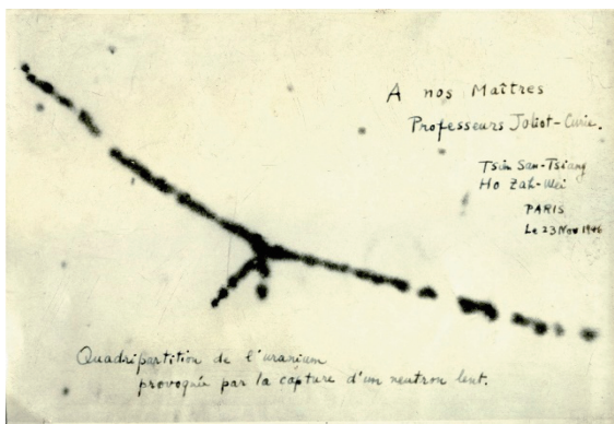
图2 钱三强、何泽慧给约里奥-居里夫妇的四分裂径迹照片
