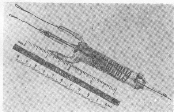
图 6. 费米小组自制的盖革计数器
