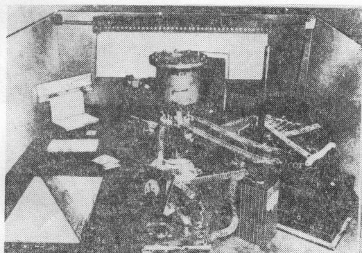
图 5. 费米小组研究慢中子用过的游离室和静电计
