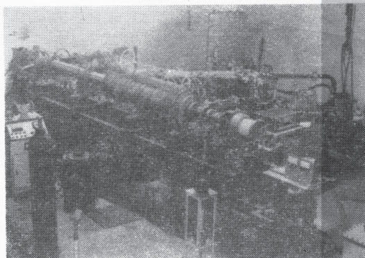
2. 30 MeV 直线加速器
