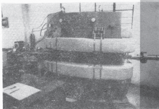
4. 储存环弯段真空室
