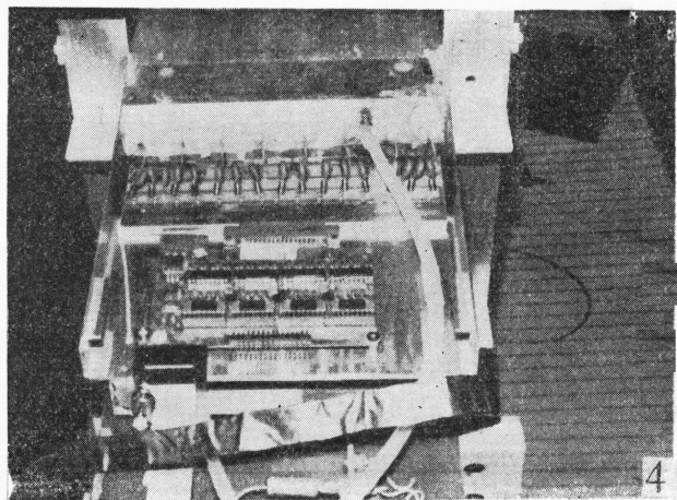
4、高能物理所与美国 MIT 合作研制出 \mu 探测器单元模型端部结构
