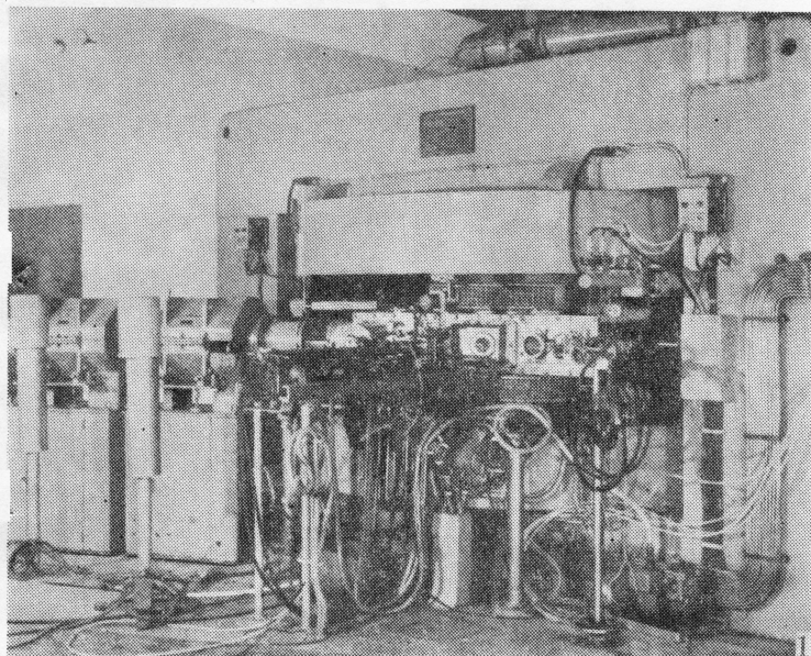
1. H-120 回旋加速器
