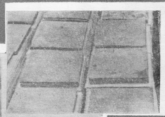
←今年八月建成的 5.2 平方米厚乳胶室和 8.5 平方米薄乳胶室及其内部构造
