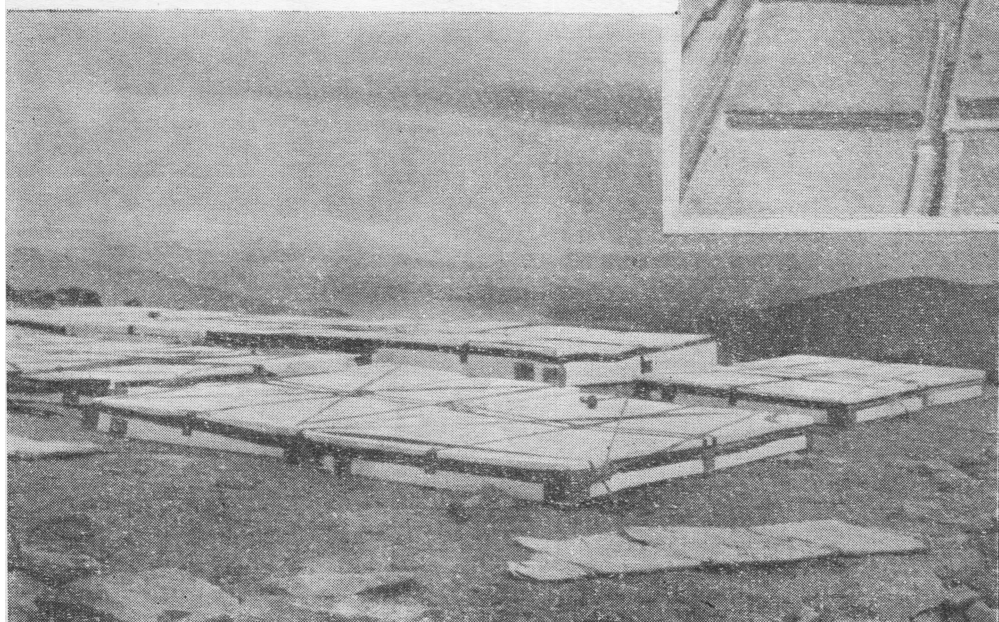
←今年八月建成的 5.2 平方米厚乳胶室和 8.5 平方米薄乳胶室及其内部构造
