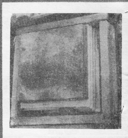
一九七六年七月第一次放置在山上的 0.3 平方米乳胶室的内部构造
