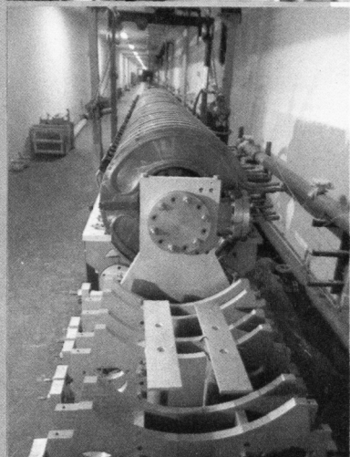
安装在隧道中的直线加速部分
