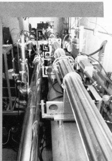
90兆电子伏电子直线加速器
