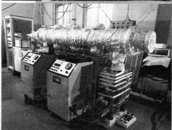
二极磁铁与四极磁铁 静电分离器进行超高真空试验
