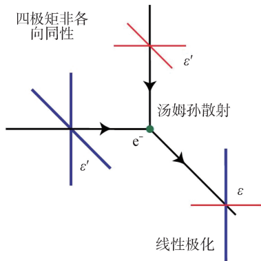
图 4 有四极矩的自然光散射后成为偏振光 (图片来源于网络 Wayne Hu 主页)
