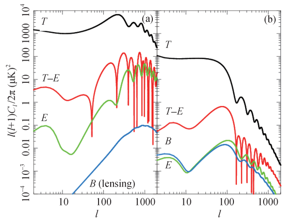
图 6 标量扰动 (a) 和引力波 (b) 产生的 CMB 角功率谱 (图片来源于网络 Challinor & Peiris, arXiv: 0903.5158)
