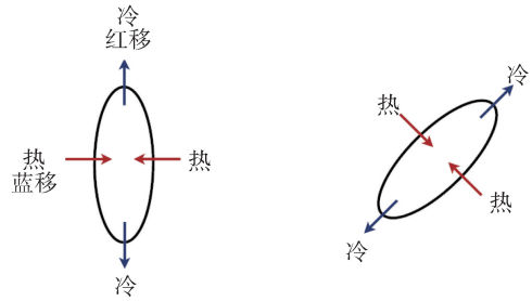
图 5 引力波独立偏振模式及其效应
