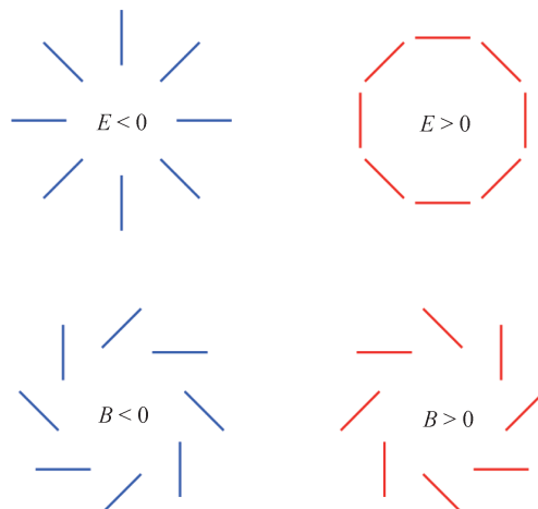
图 3 E 模式和 B 模式的偏振图像
