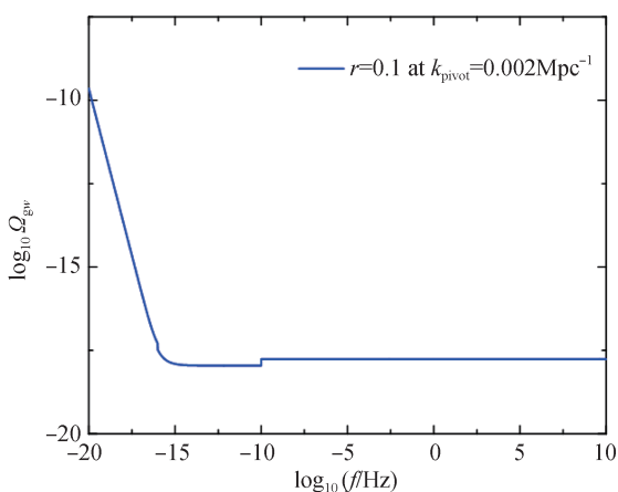
图 2 原初引力波的能量谱
