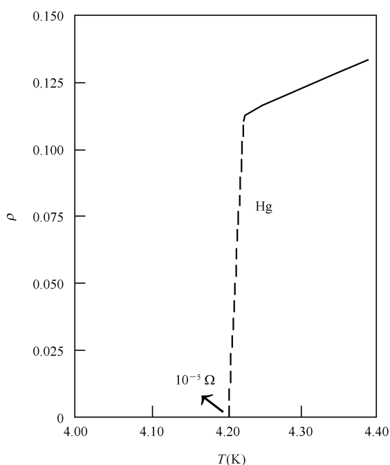
图1 超导体的正常态-超导态转变
