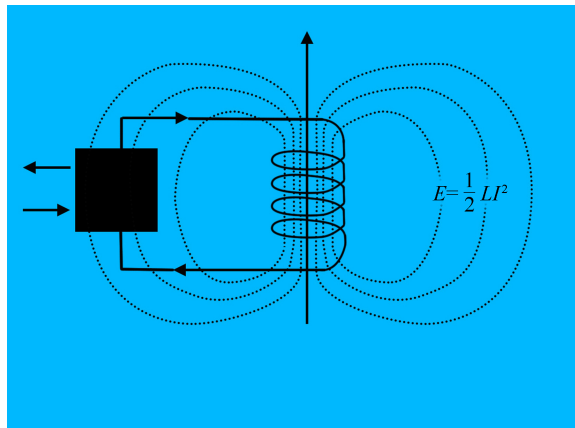
图5 超导储能系统的基本原理
