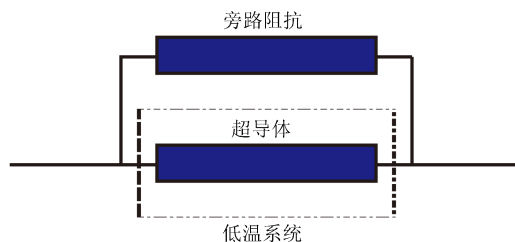
图4 超导限流器的基本原理
