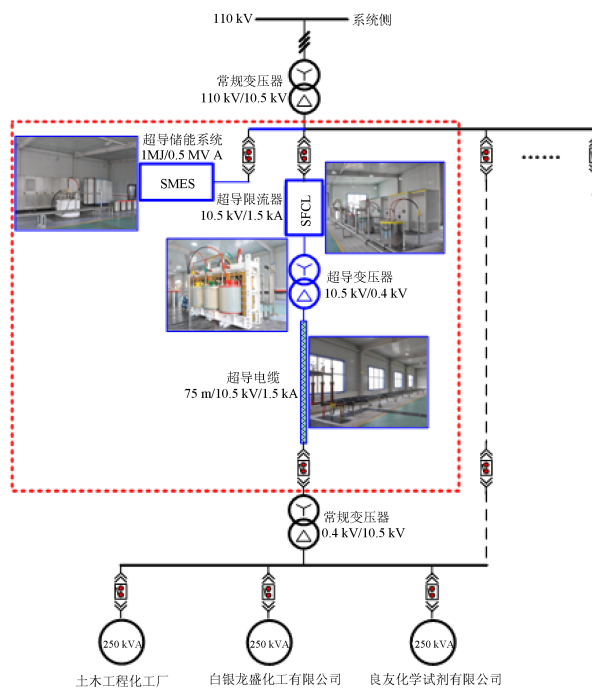
图 7 国际首座示范性超导变电站的结构示意图
