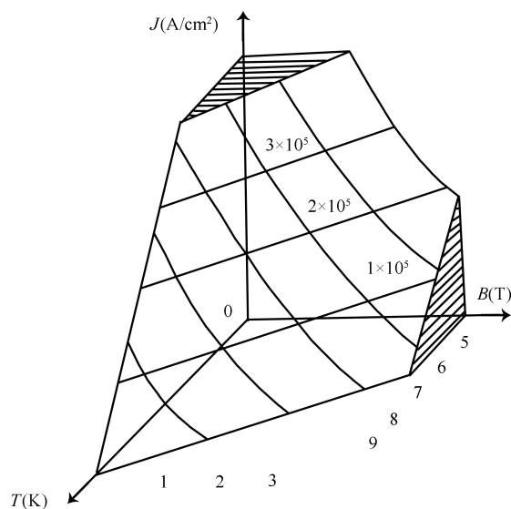
图2 超导体三个临界参数及其相互关系
