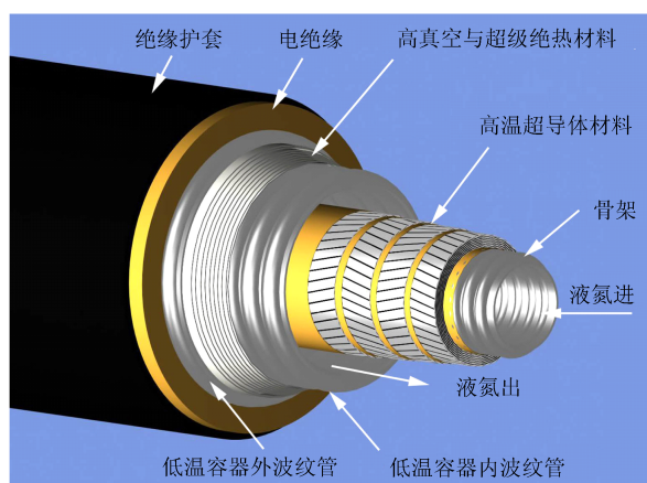
图 6 一种超导电缆的结构图
