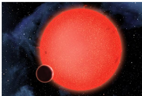
GJ1214b 想象图
