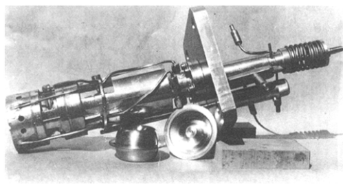
图 2 世界第 1 个速调管照片
