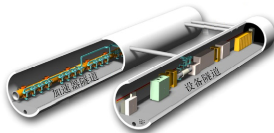
图 7 ILC 断面效果示意图
