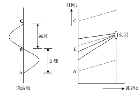
图 3 速度调制原理示意图
