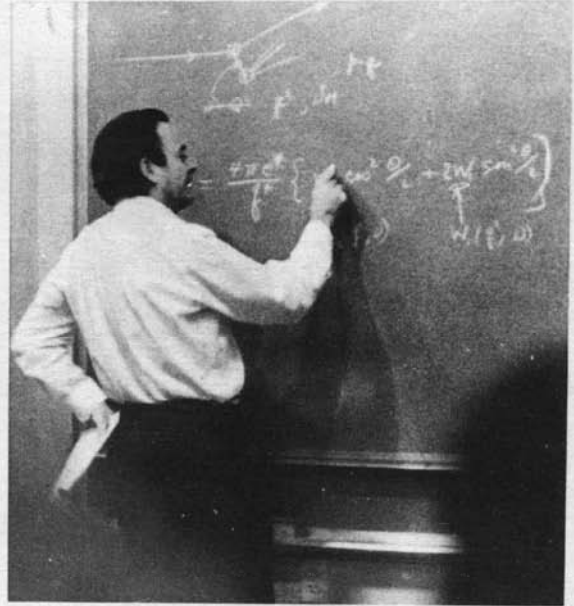
↑ 1968年10月费因曼正在用部分模型解释电子质子深度非弹性散射的实验结果。
