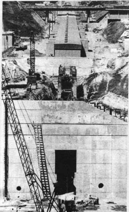
↑ SLAC 2英里长电子直线加速器的隧道工程。
