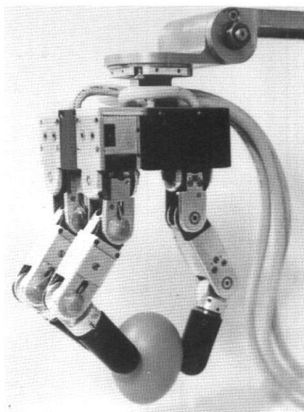
三指灵巧手,图中所持为一生鸡蛋
