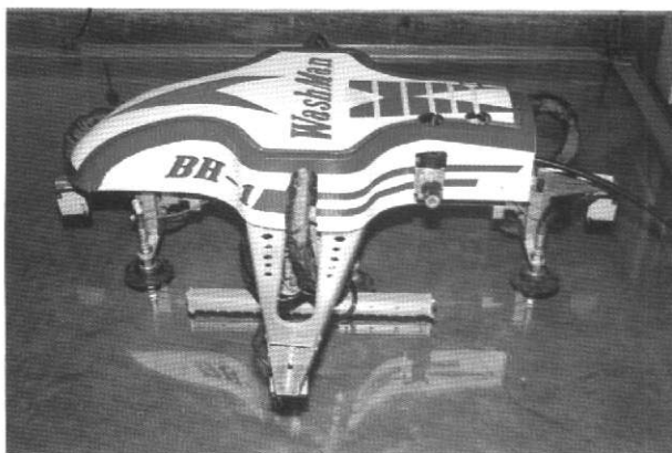
擦窗机器人,可用于擦洗高大建筑的玻璃幕墙
