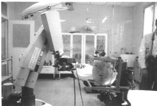
立体定向脑外科机器人集成系统。可辅助医生进行手术
